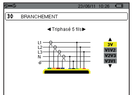
Figure 16 : connexion en triphasé 5 fils
