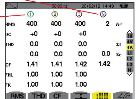
Figure 80 : l'écran affichage simultané en 4A
