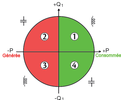
Figure 123 : diagramme des 4 quadrants
