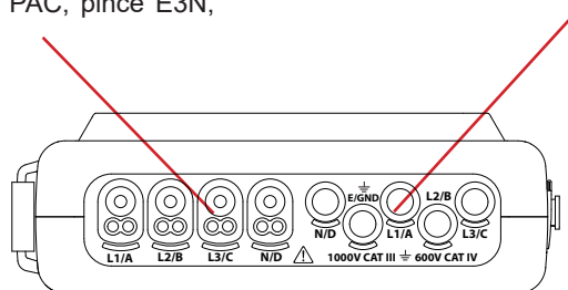
Figure 3 : les bornes de branchement
