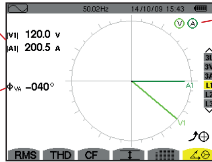
Figure 83 : l'écran d'affichage du diagramme de Fresnel en L1
