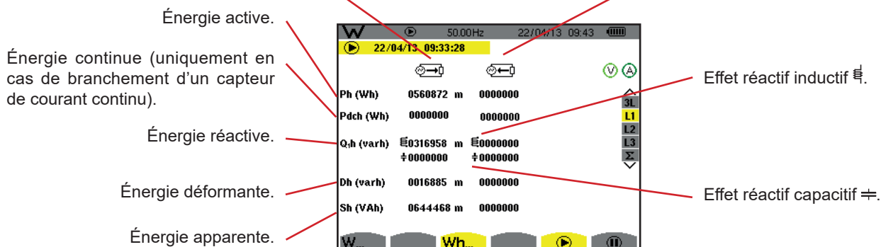
Figure 114 : l'écran d'affichage énergies consommées et générées en L1
