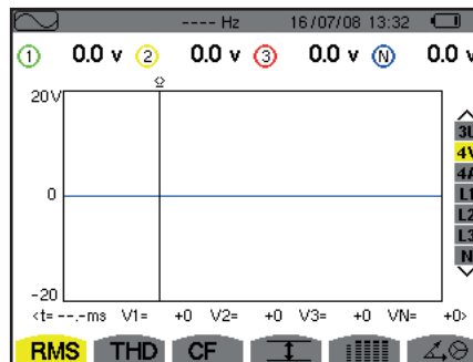
Figure 7 : l'écran Formes d'onde
