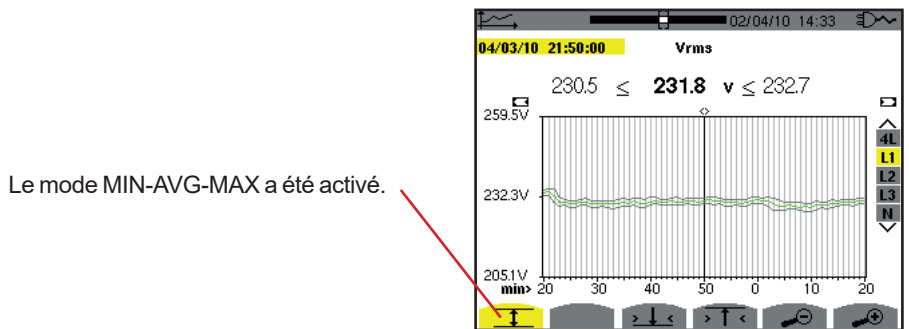
Figure 96 : Vrms (L1) avec MIN-AVG-MAX
