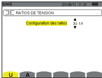
Figure 26 : l'écran Ratios de tension dans le menu Capteurs et ratios dans le cas d'un montage sans neutre
