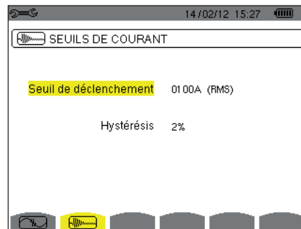
Figure 30: l'écran Seuils de courant d'appel dans le menu Mode courant d'appel
