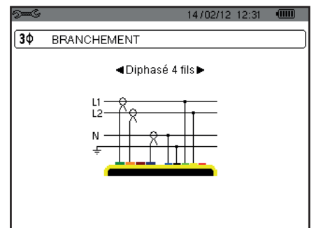
Figure 13 : connexion en diphasé 4 fils
