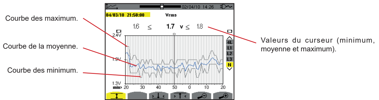
Figure 94 : Vrms (N) avec MIN-AVG-MAX
