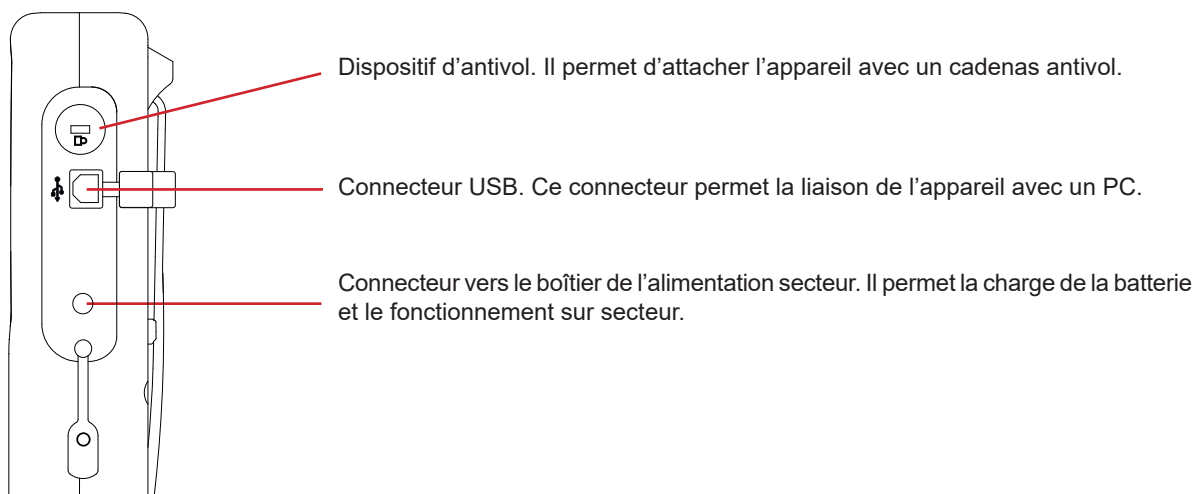
Figure 4 : les connecteurs latéraux
