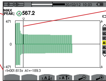
Figure 50 : l'écran d'affichage PEAK en A1 pour un branchement triphasé sans neutre
