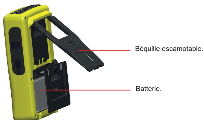
Figure 5 : béquille et trappe d'accès à la batterie
