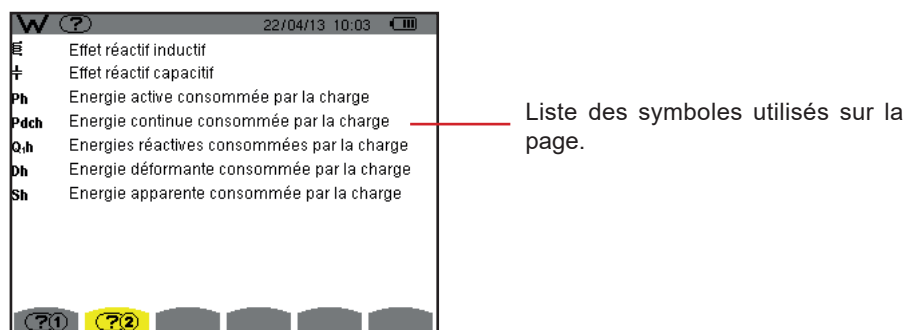
Figure 122 : l'écran de la page d'aide pour le mode puissances et énergies, page 2
