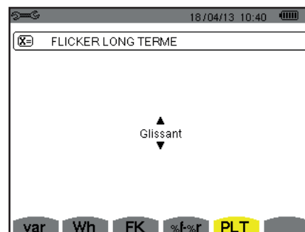
Figure 24 : le menu Choix de la méthode de calcul du PLT
