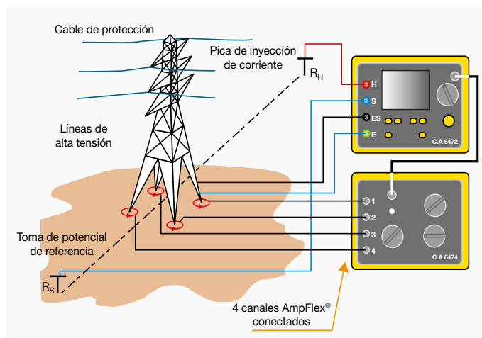
Medida de tierra del poste con los C.A 6472 + C.A 6474
